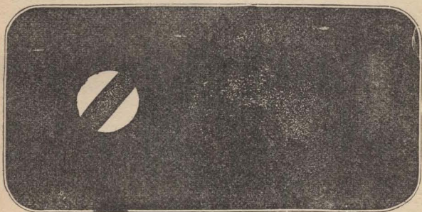
Mercurio comparado con la Tierra.
